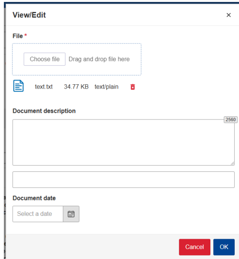
圖 19 上傳附件
