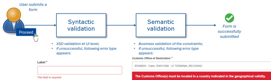
圖 9 表單驗證
